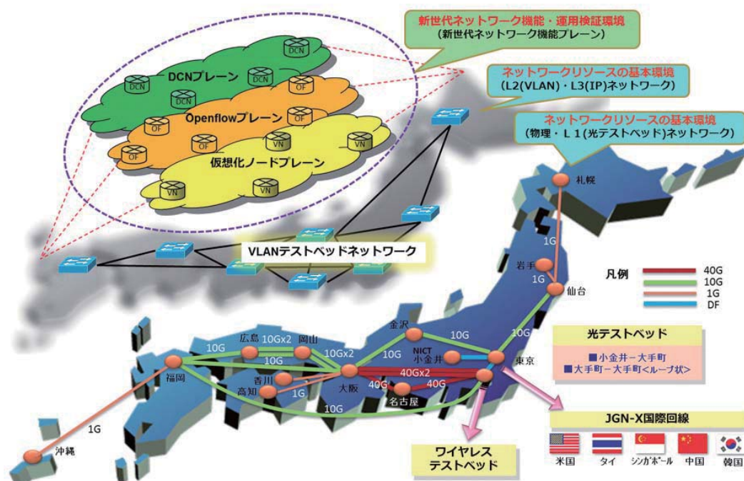
平成 26 年 1 月現在の JGN-X ネットワーク構成 (出展元:「JGN-X」Web サイトより)
